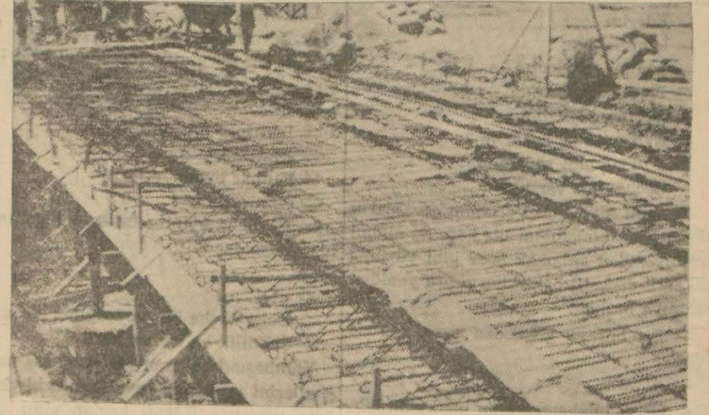
Açılacak kanallar üzerinde yapılmakta olan bir köprü
